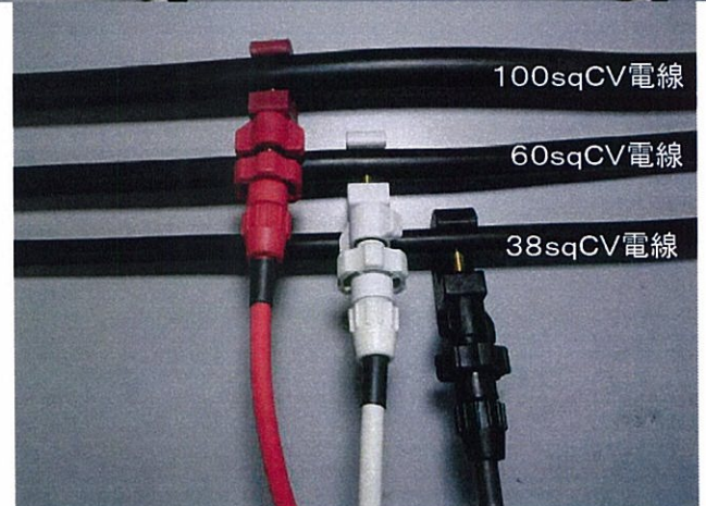
接続端子及びリード線セット
